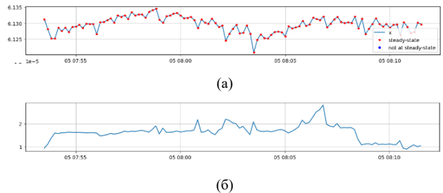
Рис. 3. Определение граничного значения величины R . а) Стационарный участок изменения параметра; б) Определение максимального граничного значения R на стационарном участке
