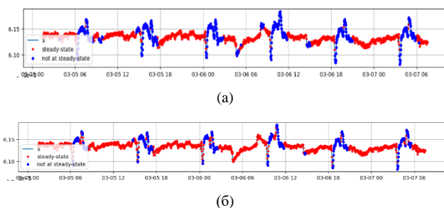
Рис. 5. Результаты идентификации стационарных режимов: а) с подобранными коэффициентами веса ( \lambda_1=0,271 , \lambda_2=0,198 , \lambda_3=0,132 ); б) без подбора коэффициентов веса ( \lambda_1=0,1 , \lambda_2=0,1 , \lambda_3=0,1 )
