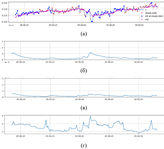
Рис. 1. Работа алгоритма по выделению стационарного режима. а) Результат работы алгоритма; б) Первая оценка дисперсии; в) Вторая оценка дисперсии; г) Отношение оценок дисперсии изменения технологического параметра
