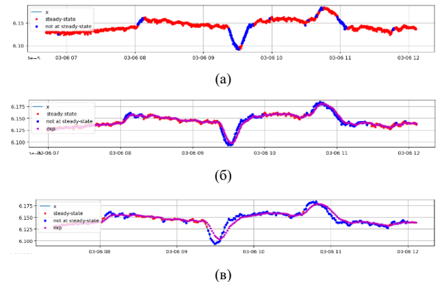
Рис. 4. Результат работы алгоритма при различных частотах дискретизации. а) частота дискретизации 1/10 \text{ c}^{-1} ; б) частота дискретизации 1/30 \text{ c}^{-1} ; в) частота дискретизации 1/60 \text{ c}^{-1}
