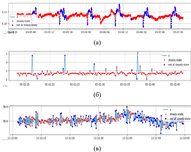
Рис. 2. Результат работы алгоритма идентификации стационарного режима для технологических параметров: а) расход; б) давление; в) температура
